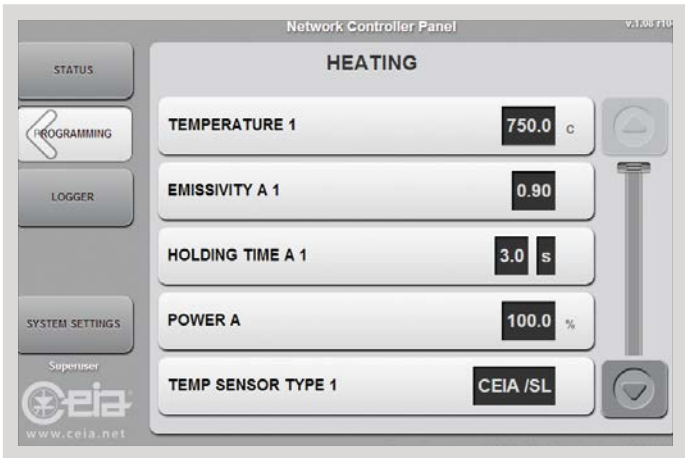
► HEATING MENU
