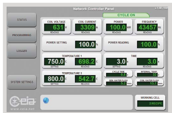
► MAIN SCREEN
