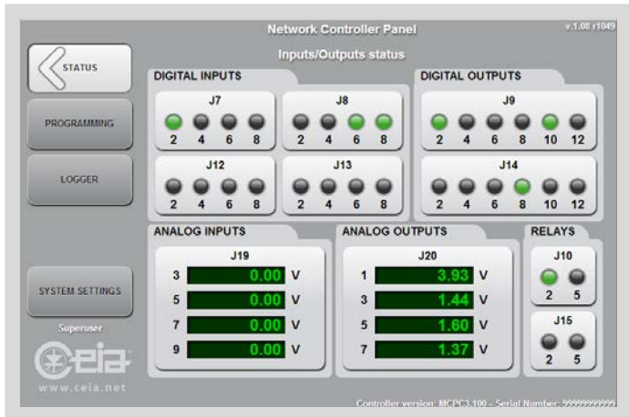
► INPUT/OUTPUT STATUS
