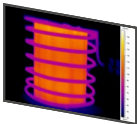
CONTROL TERMOCÁMARA
